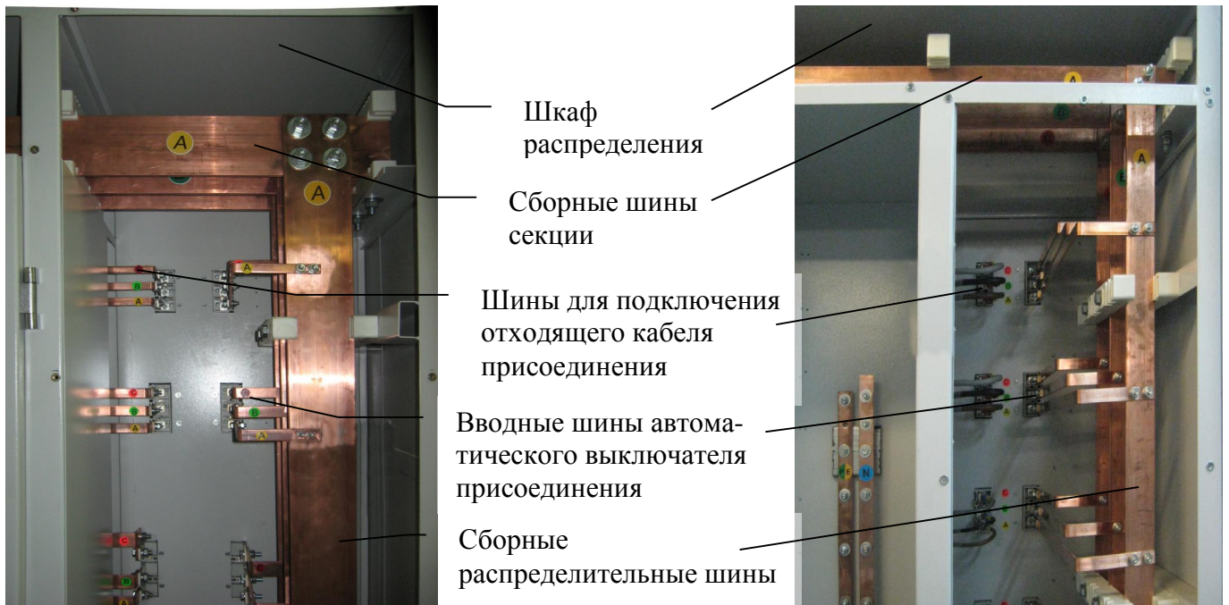
Рис. 8 Шинный отсек шкафа распределения (вид с задней стороны)
