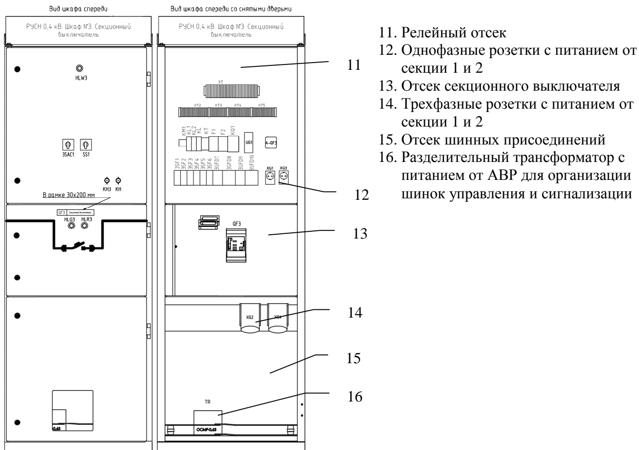
Рис. 3 Шкаф секционного выключателя.
