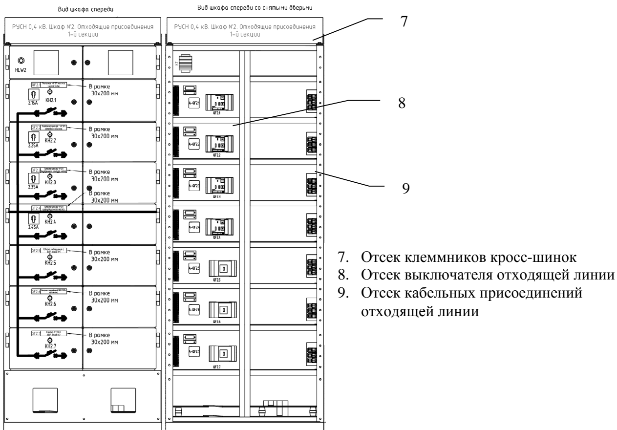
Рис. 2 Шкаф распределения.
