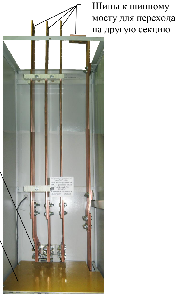
Рис. 5 Шкаф секционного выключателя НКУ-РУСН при двухрядном расположении секций
