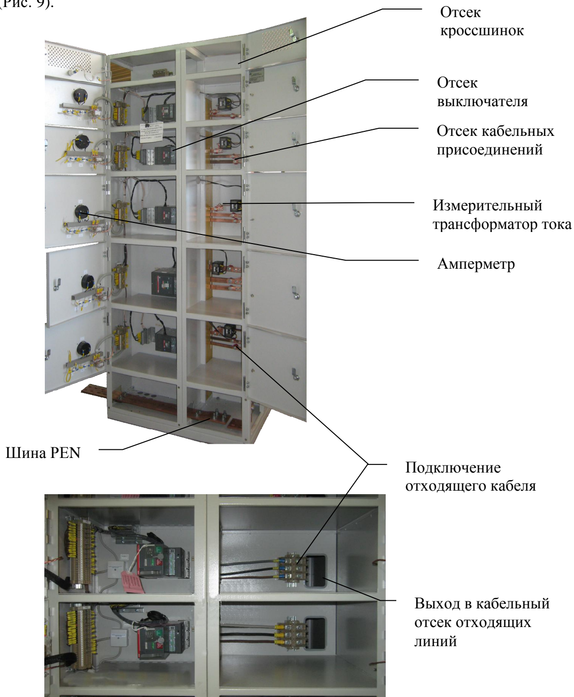
Рис. 7 Шкаф распределения НКУ-РУСН
