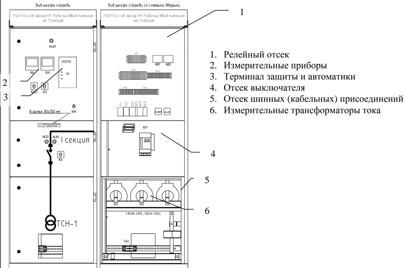
Рис. 1 Шкаф ввода .
