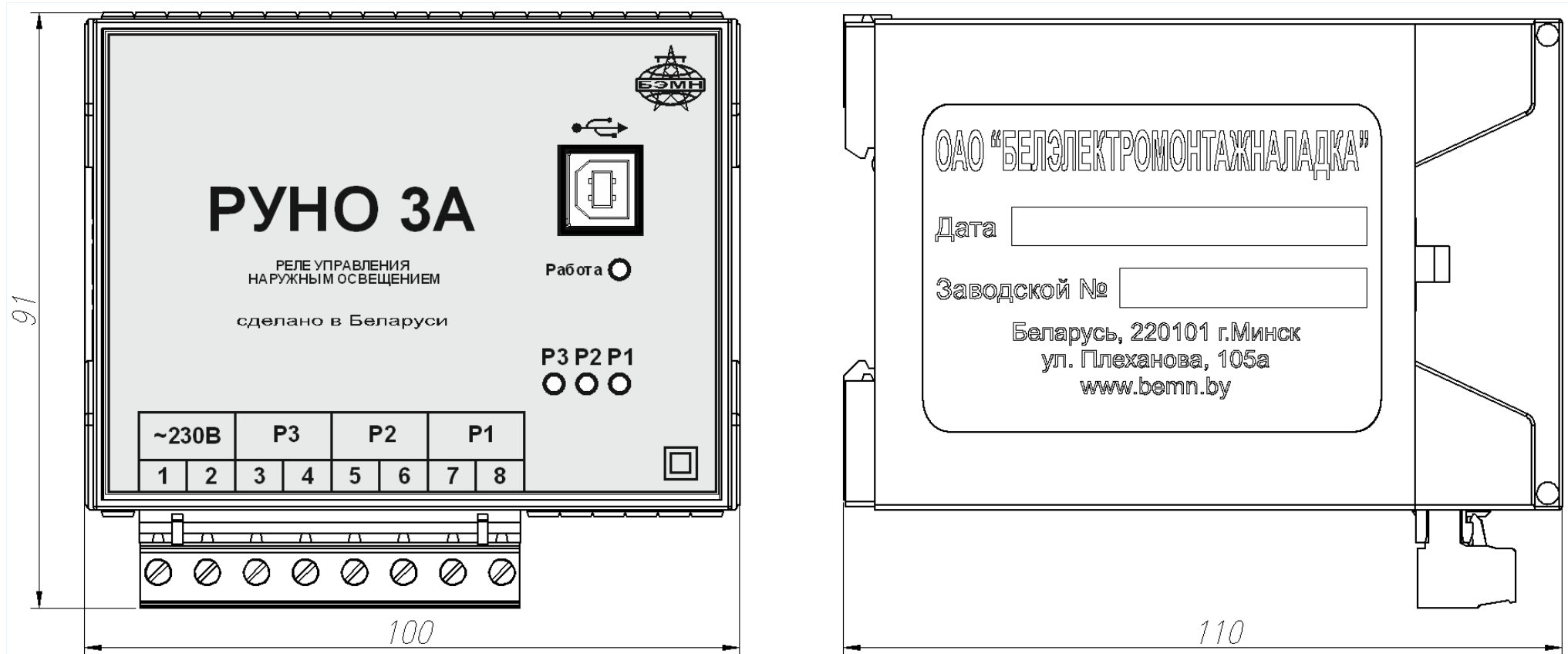
Рисунок 1 – Габаритный чертёж РУНО 3А
