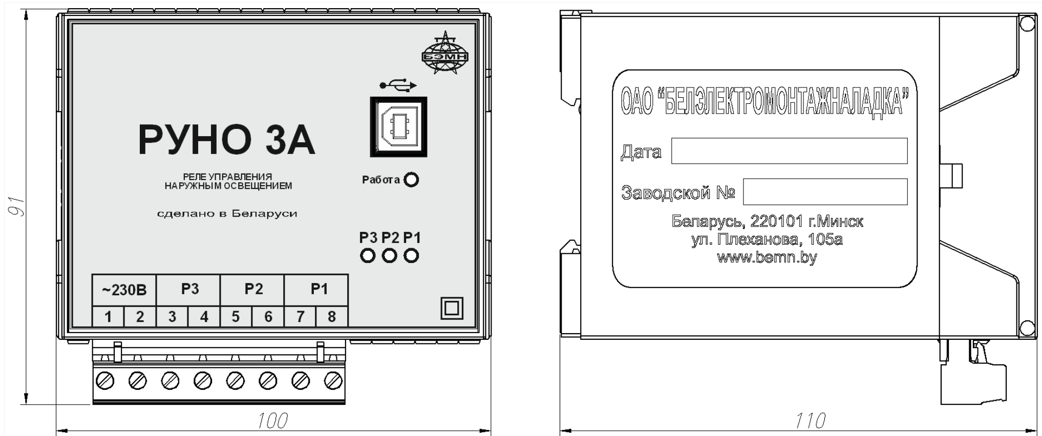
Рисунок А.2 – Габаритные размеры РУНО 3А
