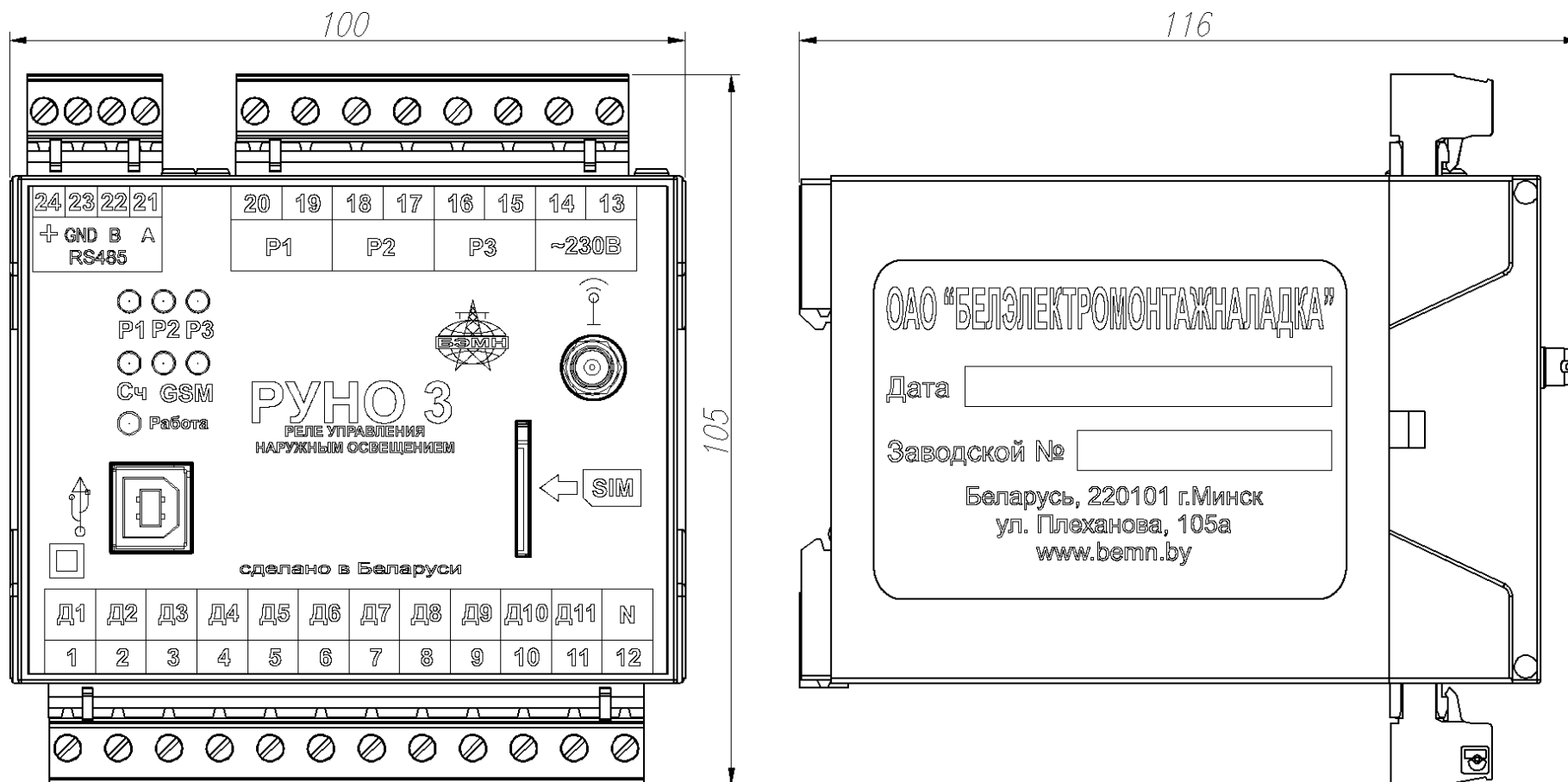
Рисунок А.1 – Габаритные размеры РУНО 3
