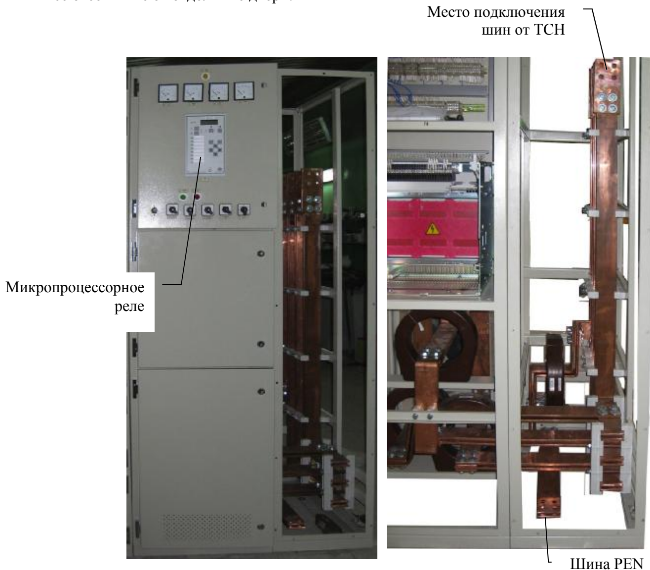
Рис. 5 Шкаф ввода и стыковочный шкаф. Лицевая сторона
