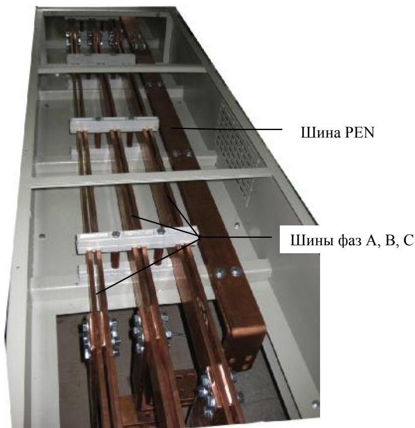
Рис. 11 Шинный мост
